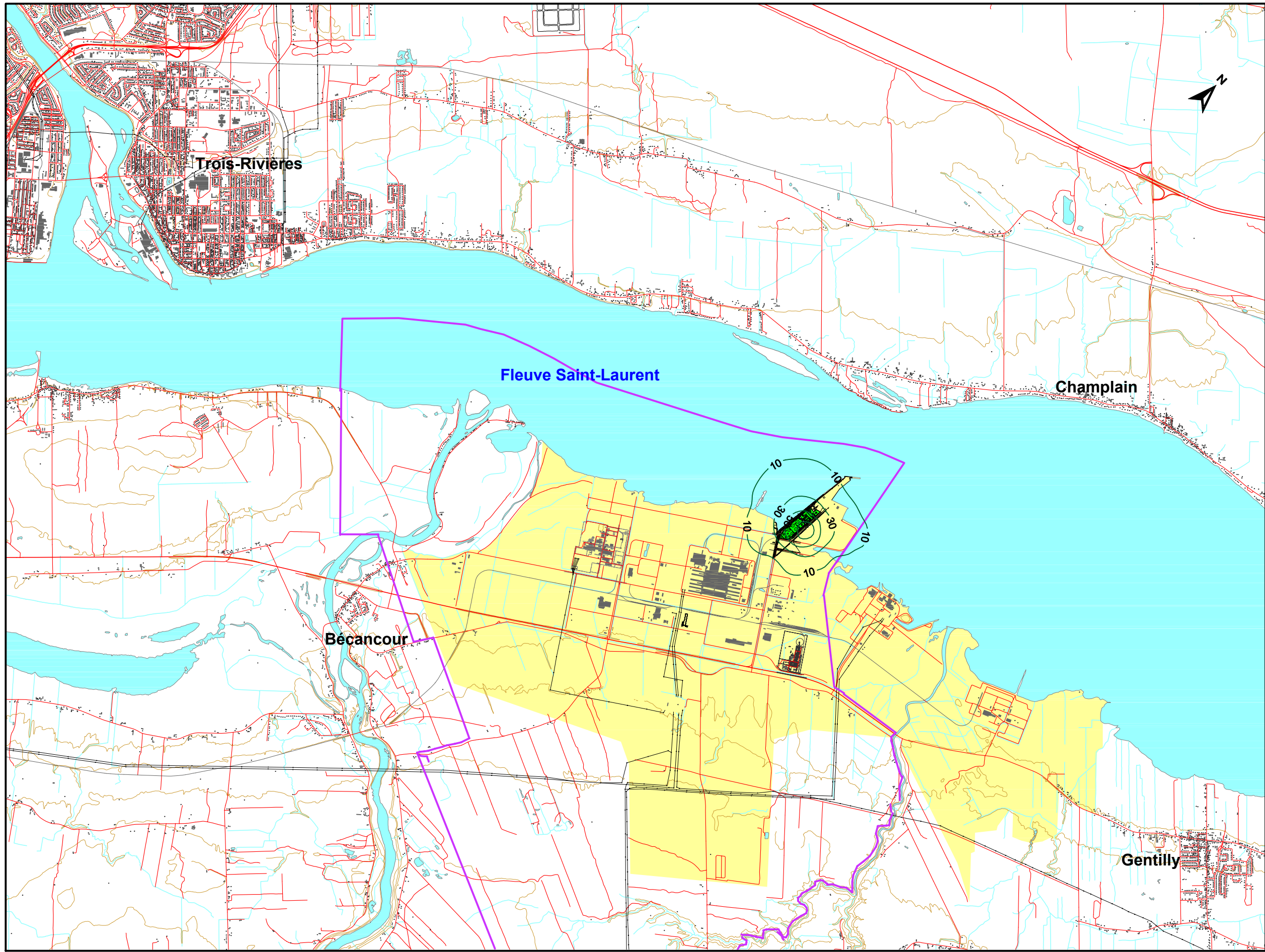
Figure 3.10 Concentrations maximales ( \mu\text{g}/\text{m}^3 ) de benzène sur une période de 24 heures, année 1999
